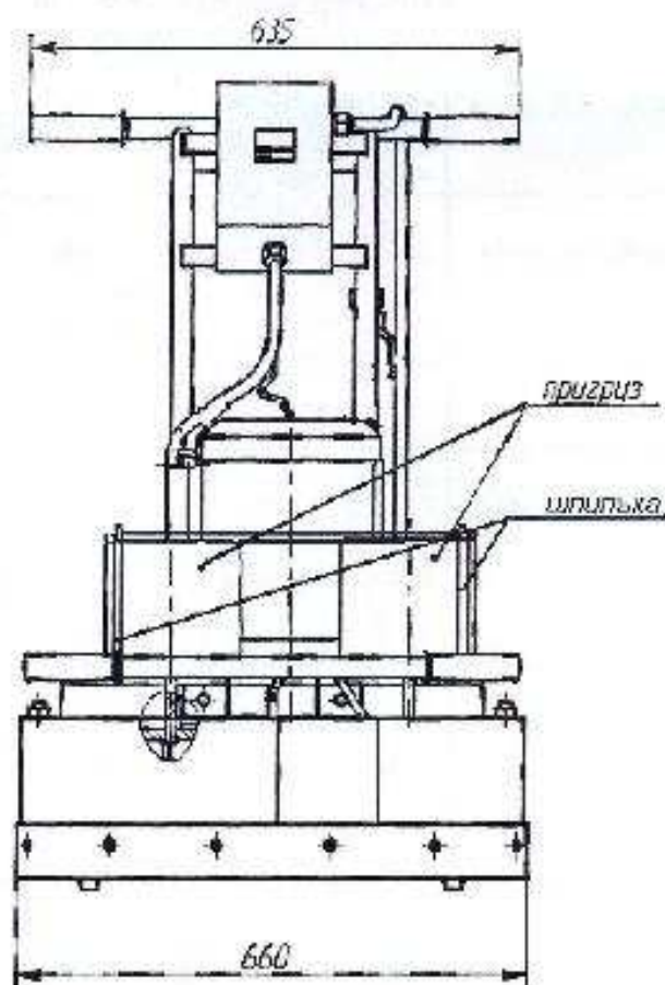
Рисунок 3 – Крепление пригрузов на машину
