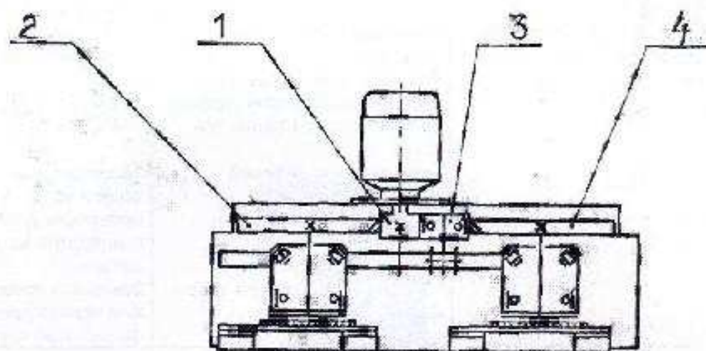
Рисунок 2 - Схема кинематическая
