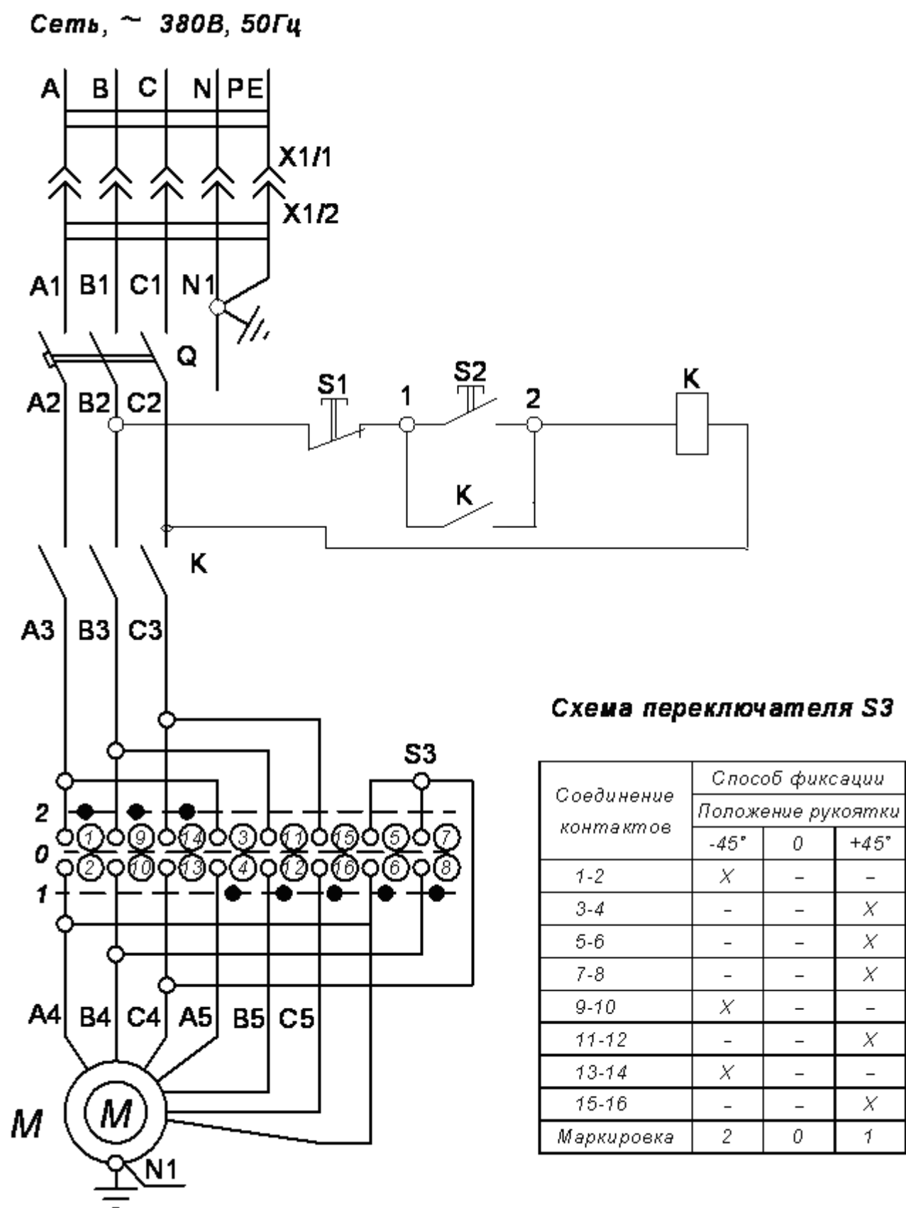
Рисунок 4 – Схема электрическая принципиальная
