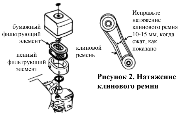
Рисунок 1. Воздушный фильтр
